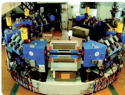
L'Anneau de Collision du LAL
