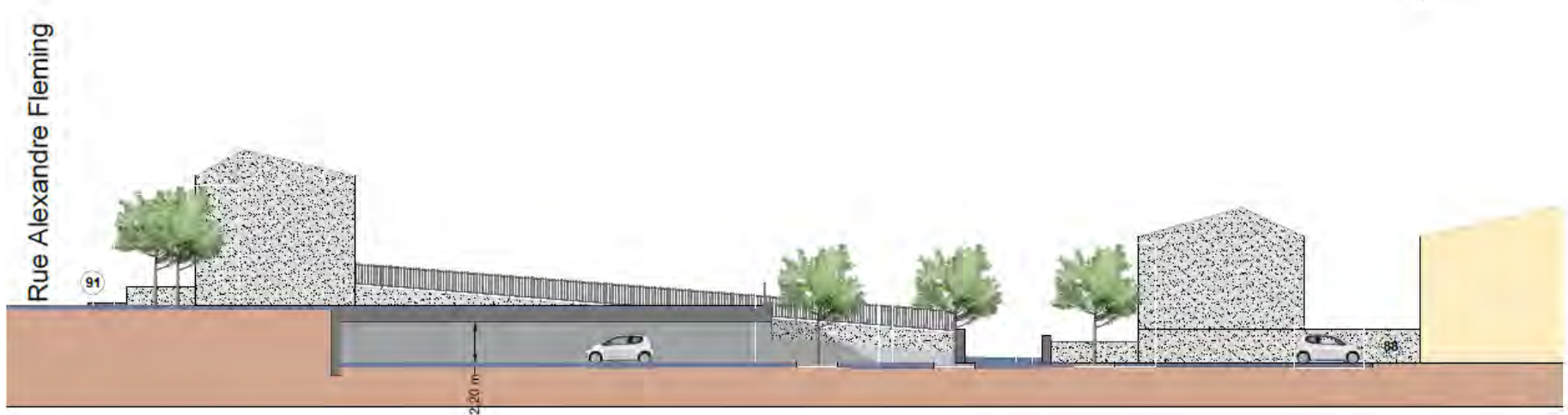
Proposition (vue en coupe) : Parking Kempen
